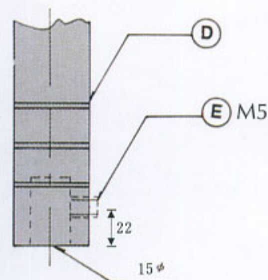
Hand Press T6精密手壓機
